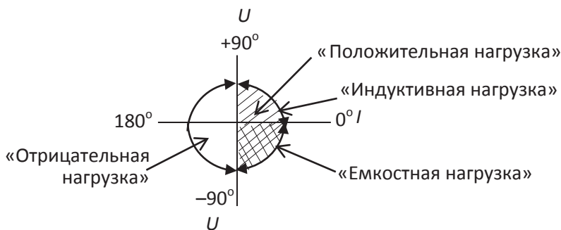
Рис. 1.1. Виды нагрузок при измерении мощности
