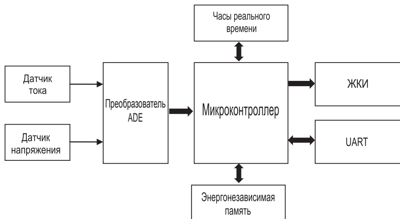
Рис. 1.6. Структурная схема однофазного счетчика ЭЭ на базе микросхем ADE
