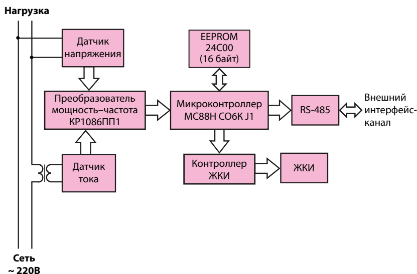
Рис. 1.4. Структурная схема простейшего однофазного счетчика ЭЭ на базе микроконтроллера МС88НС05L16
