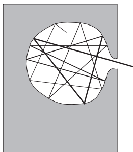
Рис. 1.1. Замкнутая полость может служить моделью абсолютно черного тела, так как попадающее в нее излучение после многократного отражения от стенок поглощается практически полностью. Макс Планк изучал распределение по энергиям в излучении черного тела, то есть внутри такой полости.
