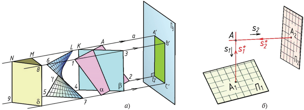
Рис. 1.4. Обратимость чертежа:
