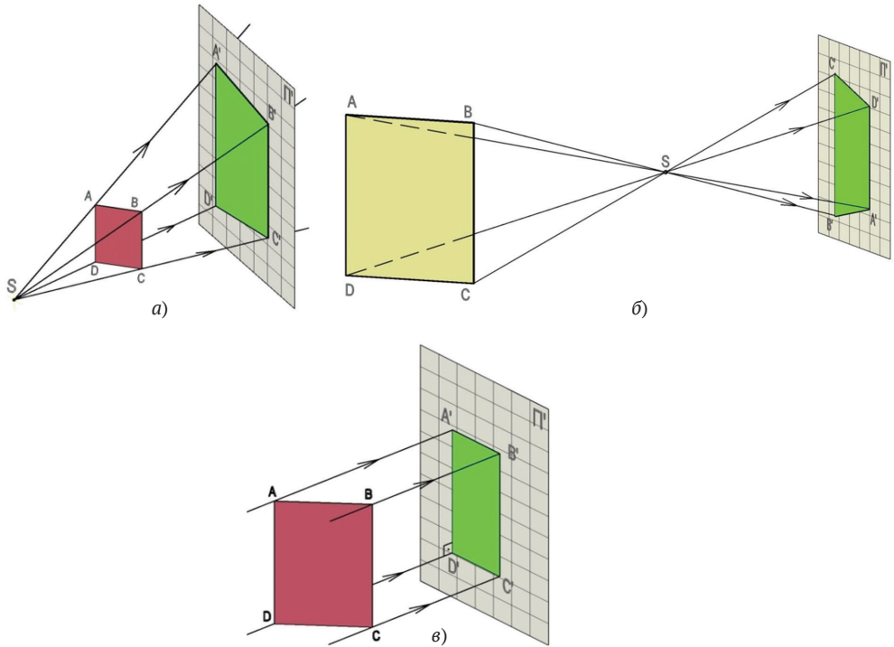
Рис. 1.3. Методы проецирования: а, б – центральное проецирование; в – ортогональное проецирование
