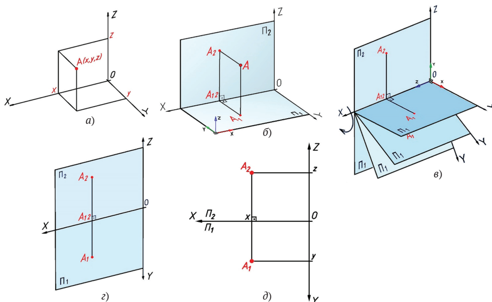
Рис. 1.5. Пространственная модель построения чертежа точки: а – точка в декартовой системе координат; б – ортогональное проецирование точки на две плоскости; в – вращение горизонтальной плоскости проекций; г – совмещение плоскостей в единую плоскость чертежа; д – чертеж точки в двух проекциях
