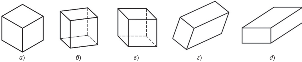
Рис. 1.13. Варианты аксонометрических проекций (на примере куба): а – ортогональная изометрия; б – ортогональная диметрия; в – косоугольная фронтальная диметрия; г, д – другие косоугольные проекции – триметрии
