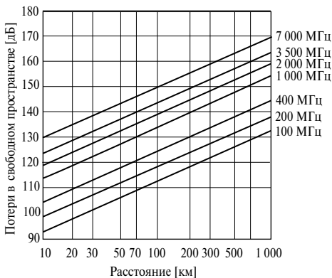
Рис. 1.5. Зависимость потерь энергии в свободном пространстве от расстояния и частоты
