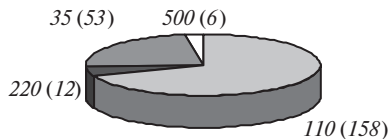
Рис. 1.1. Количество установленных трансформаторов в системе энергетики Чувашской Республики в зависимости от класса напряжения.
