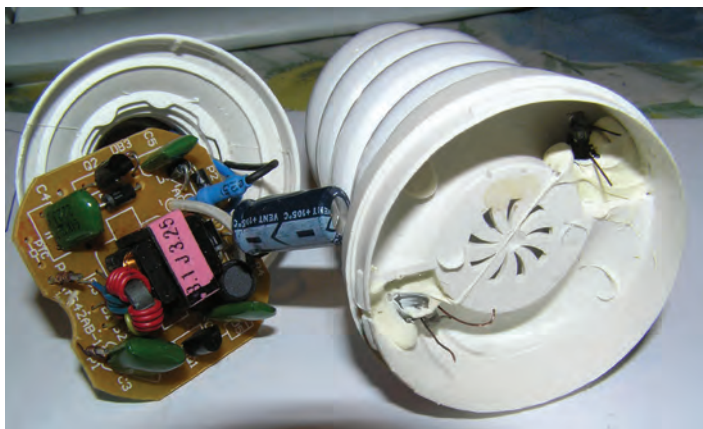
Рис. 1.4. «Начинка» энергосберегающей лампы
