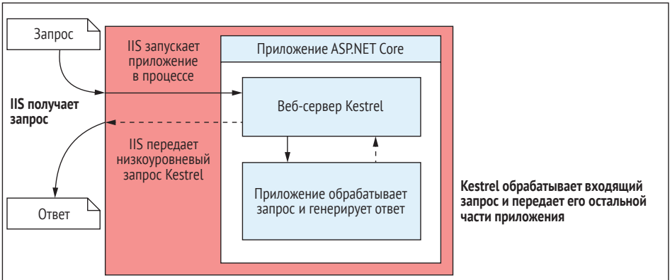
Рис. 1.7 Разница между моделями размещения в ASP.NET (вверху) и ASP.NET Core (внизу). В предыдущей версии ASP.NET IIS тесно связан с приложением. Модель размещения в ASP.NET Core проще; IIS передает запрос на локальный веб-сервер в приложении ASP.NET Core и получает ответ, но не имеет более детального представления о приложении
