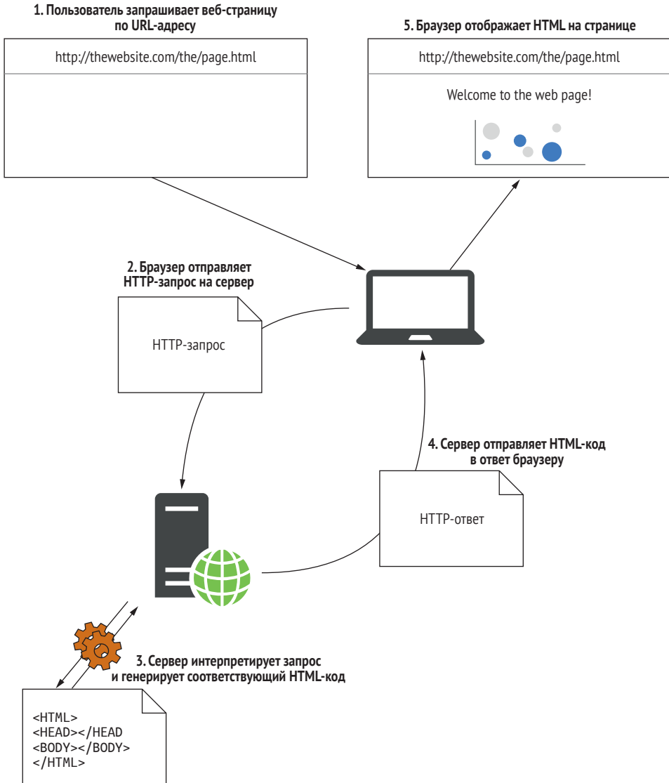
Рис. 1.8 Запрос веб-страницы. Пользователь начинает с запроса веб-страницы, что вызывает отправку HTTP-запроса на сервер. Сервер интерпретирует запрос, генерирует необходимый HTML и отправляет его обратно в HTTP-ответе. Затем браузер может отобразить веб-страницу
