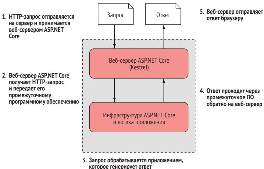
Рис. 1.9 Как приложение ASP.NET Core обрабатывает запрос. Приложение ASP.NET Core получает запрос и запускает собственный веб-сервер. Веб-сервер обрабатывает запрос и передает его телу приложения, которое генерирует ответ и возвращает его веб-серверу. Веб-сервер отправляет этот ответ браузеру
