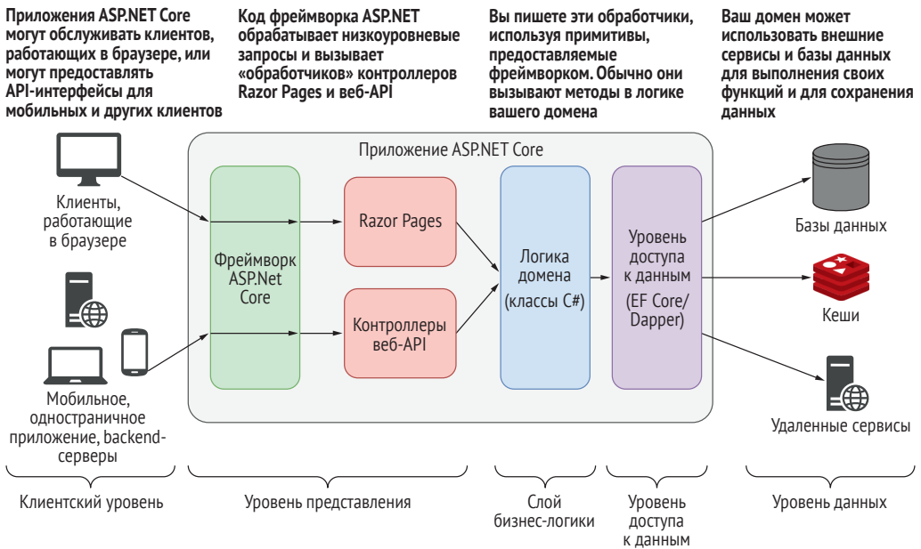
Рис. 1.1 Типичное приложение ASP.NET Core состоит из нескольких уровней. Код фреймворка ASP.NET Core обрабатывает запросы от клиента, работая со сложным сетевым кодом. Затем фреймворк вызывает обработчики (Razor Pages и контроллеры веб-API), которые вы пишете с использованием примитивов, предоставляемых фреймворком. В конце эти обработчики вызывают логику предметной области вашего приложения, которая обычно представляет собой классы и объекты C# без каких-либо зависимостей, специфичных для ASP.NET Core
