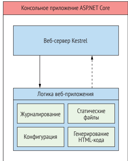
Рис. 1.4 Модель приложения ASP.NET Core. Платформа .NET 5.0 предоставляет базовую модель консольного приложения для запуска приложений командной строки. Добавляя библиотеку веб-сервера, вы преобразуете ее в веб-приложение ASP.NET Core. Дополнительные функции, такие как конфигурация и журналирование, добавляются посредством дополнительных библиотек
