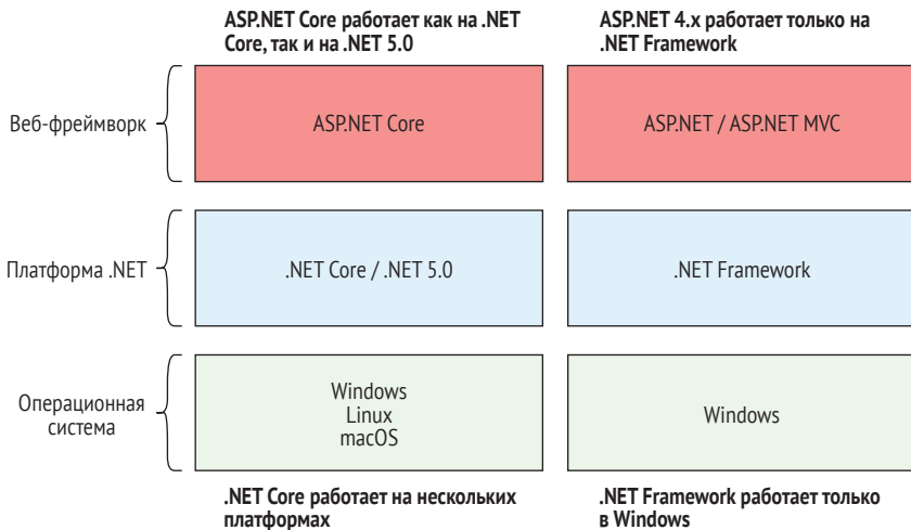
Рис. 1.3 Связь между ASP.NET Core, ASP.NET, .NET Core / .NET 5.0 и .NET Framework. ASP.NET Core работает на .NET Core и .NET 5.0, поэтому является кроссплатформенным. И наоборот, ASP.NET работает только на .NET Framework, поэтому она привязана к ОС Windows
