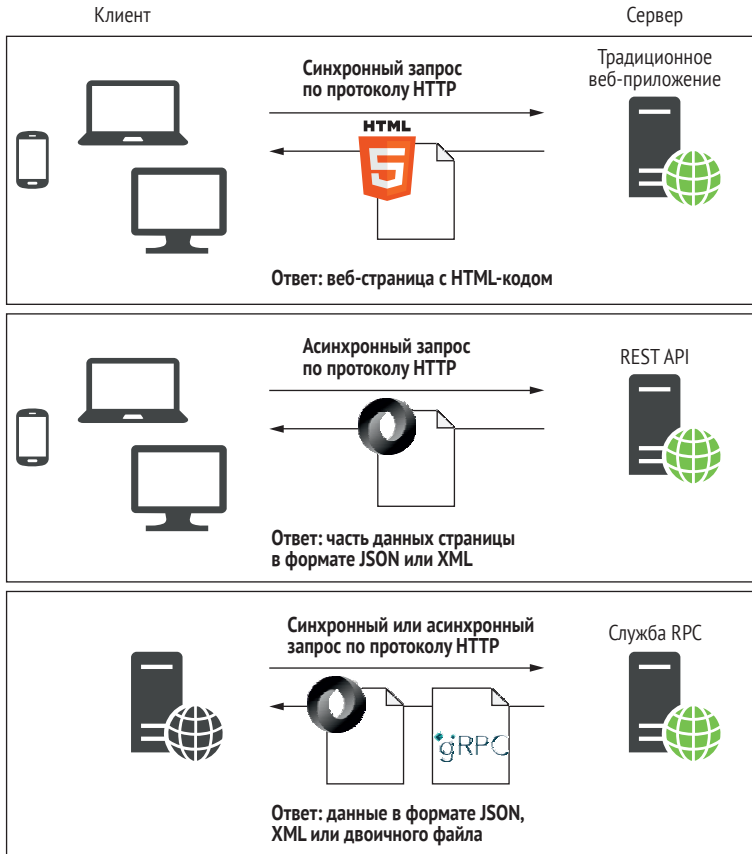
Рис. 1.6 ASP.NET Core может выступать в роли серверного приложения для различных клиентов: он может обслуживать HTML-страницы для традиционных веб-приложений, действовать как REST API для клиентских односторонних приложений или выступать в качестве специальной службы RPC для клиентских приложений
