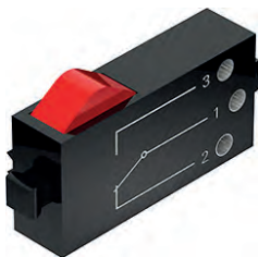
Рис. 1.9. Кнопочный переключатель
